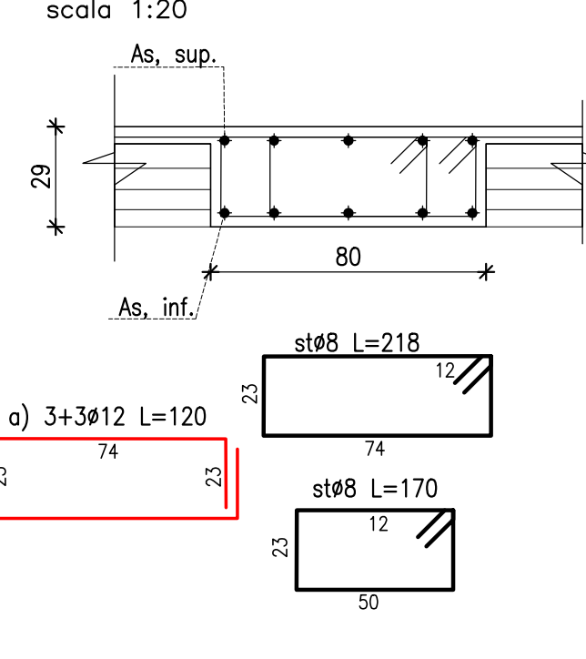
SEZIONE scala 1:20
