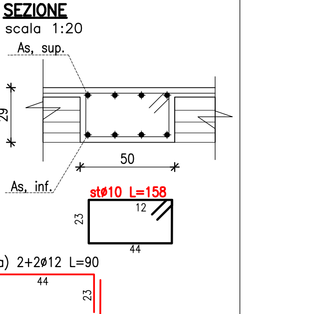
SEZIONE scala 1:20
