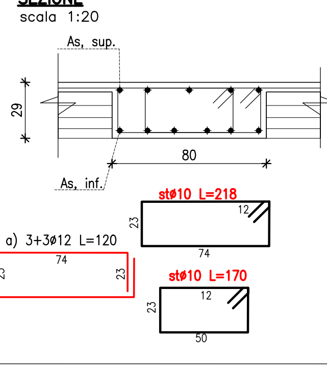
SEZIONE scala 1:20
