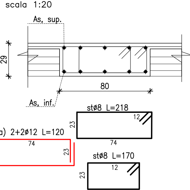
SEZIONE scala 1:20
