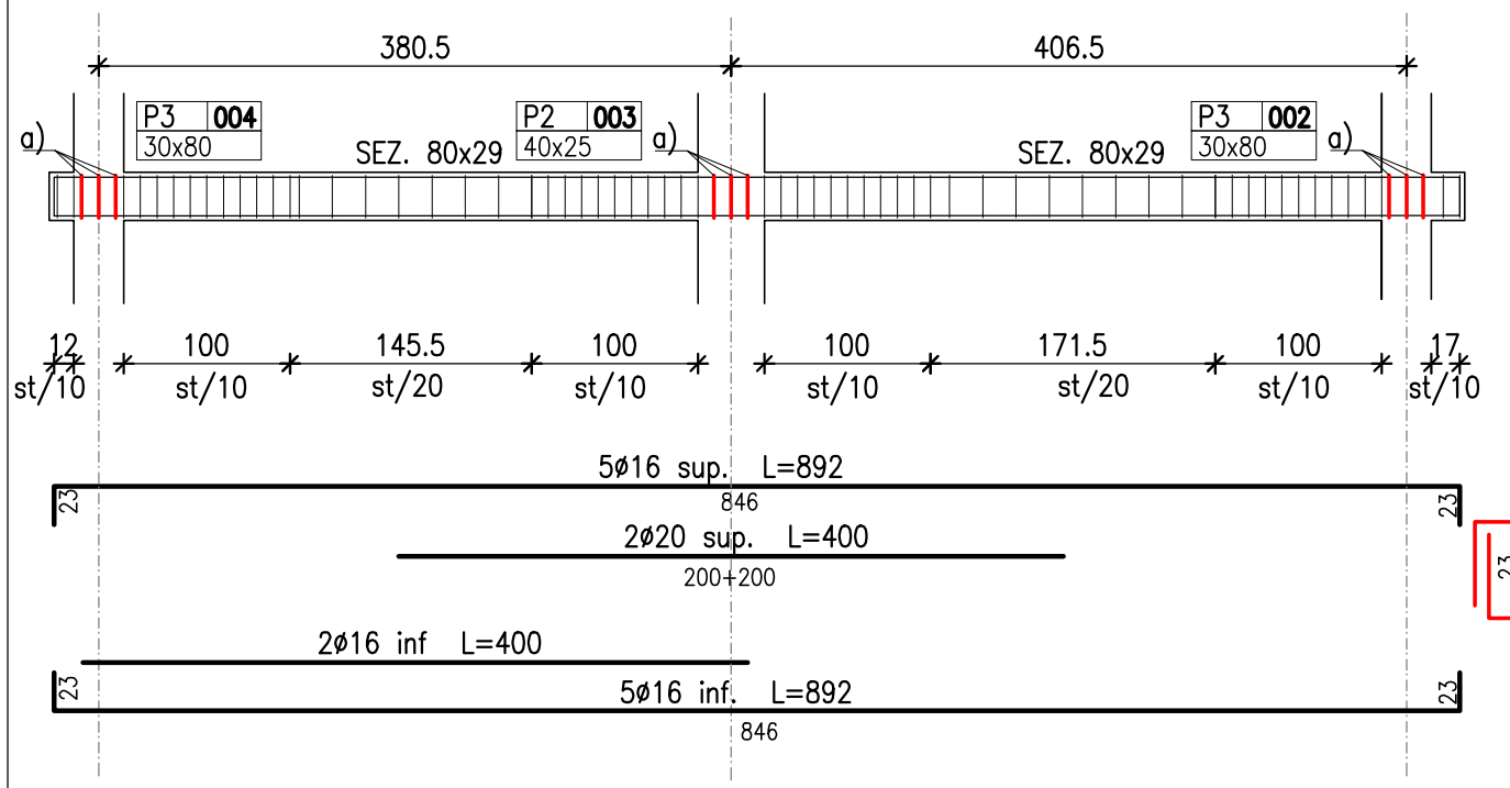
TRAVE T5 scala 1:50
