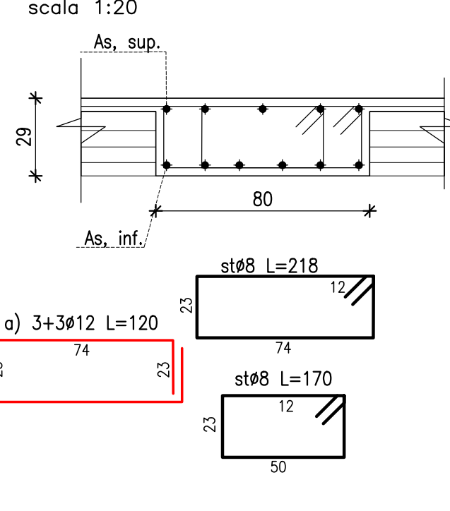
SEZIONE scala 1:20
