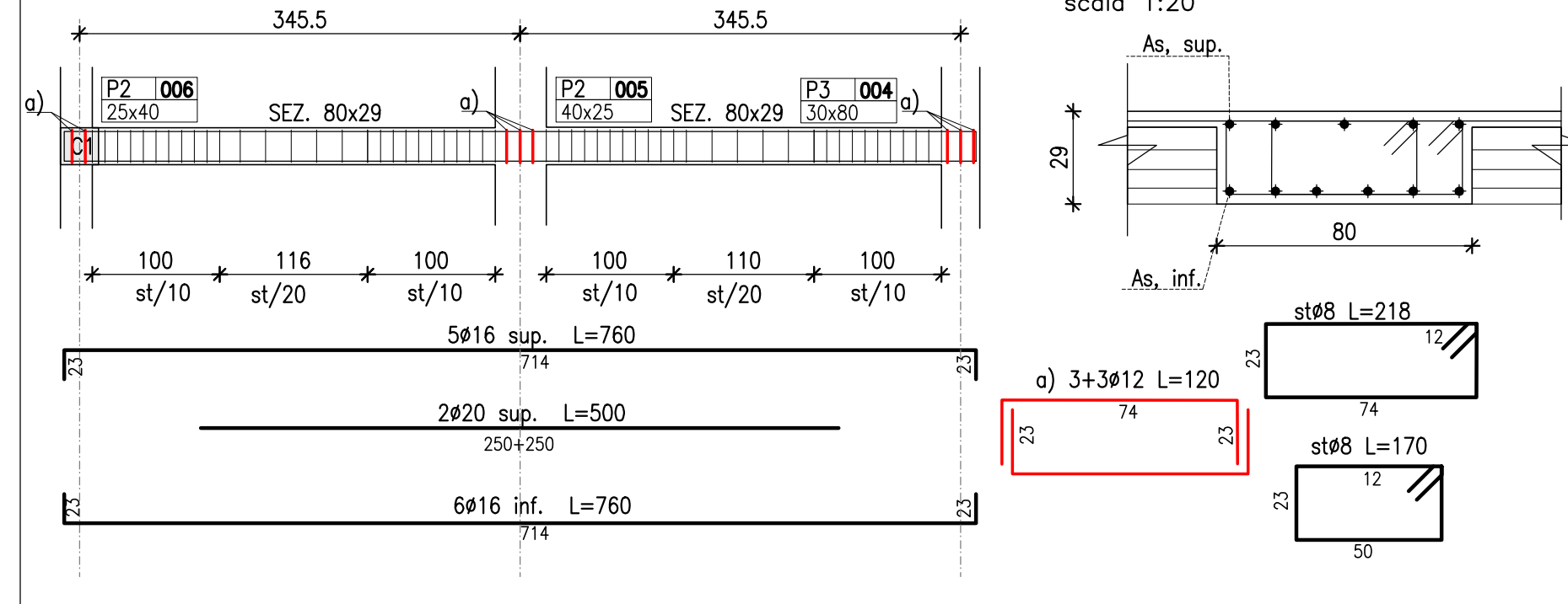
TRAVE T6 scala 1:50
