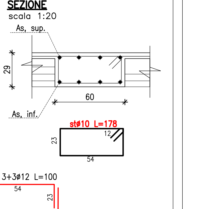
SEZIONE scala 1:20
