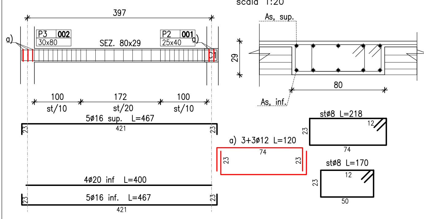
TRAVE T4 scala 1:50
