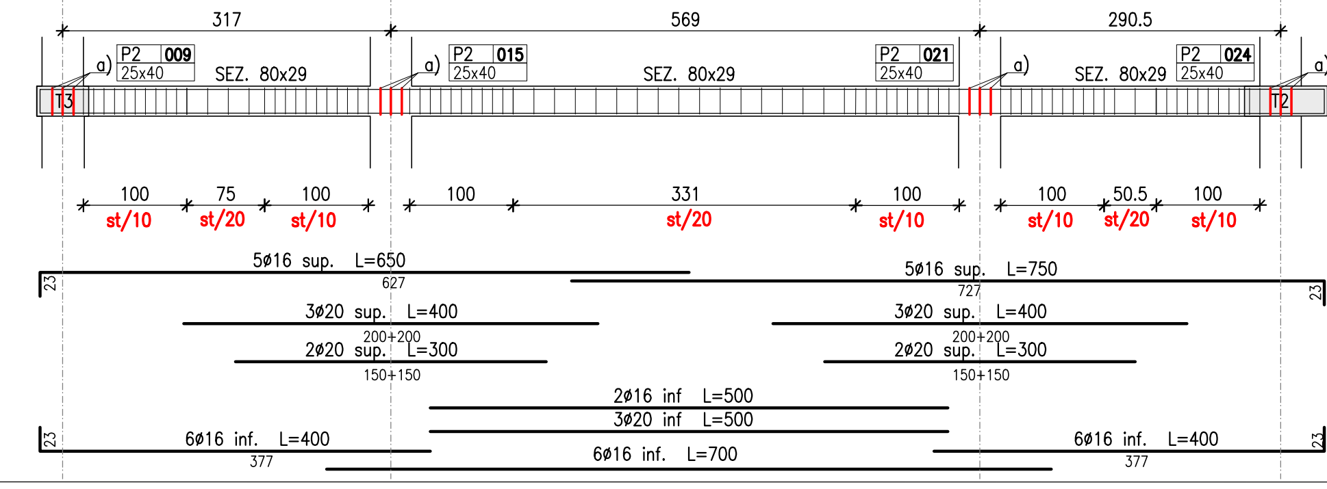
TRAVE T10 scala 1:50
