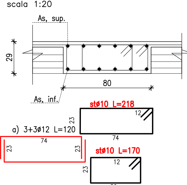
SEZIONE scala 1:20
