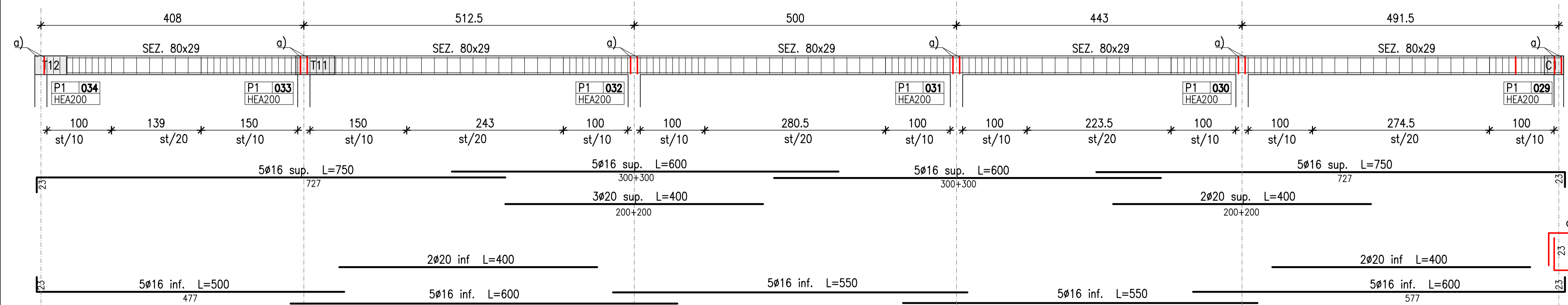
TRAVE T1 scala 1:50
